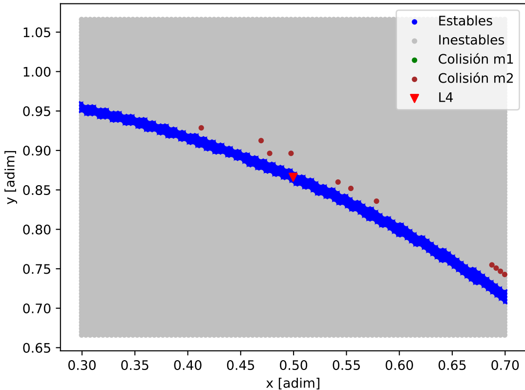
Mapa de estabilidad - HD_83443
