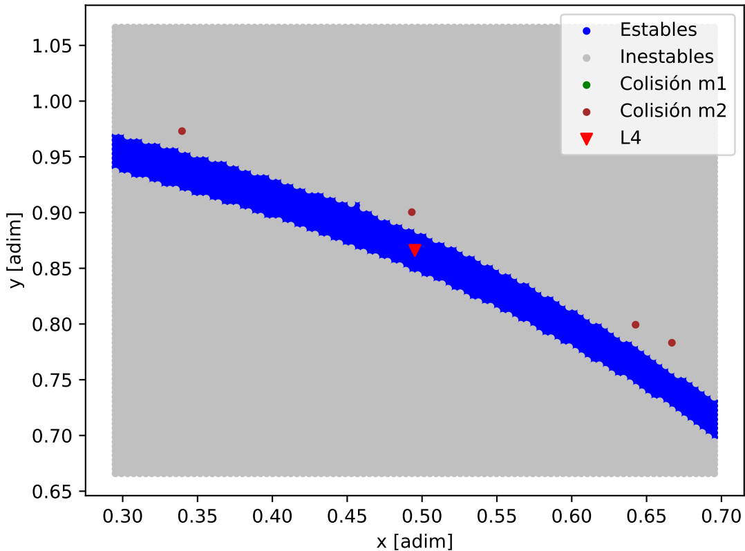
Mapa de estabilidad - HD_87816
