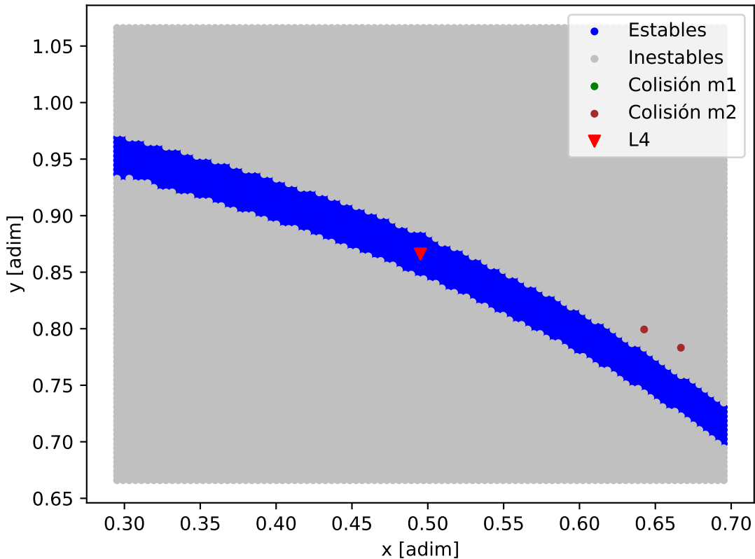
Mapa de estabilidad - HD_94890
