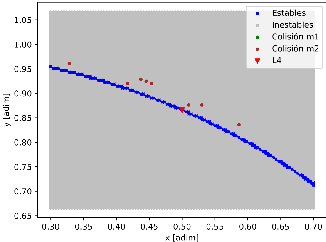
Mapa de estabilidad - HD_99492
