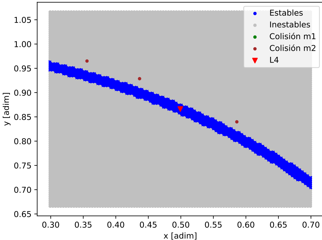
Mapa de estabilidad - HD_99706
