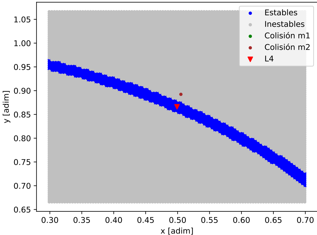
Mapa de estabilidad - HIP_111909
