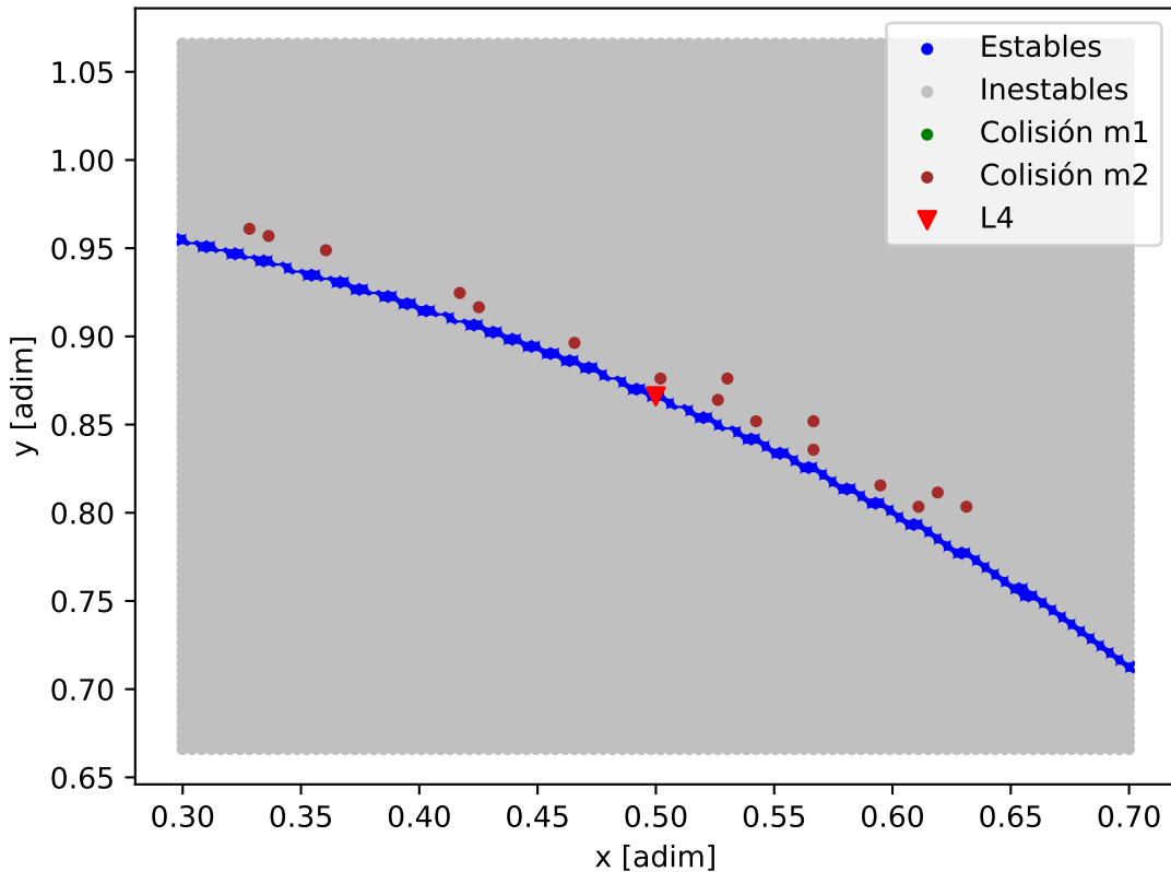
Mapa de estabilidad - HIP_54373
