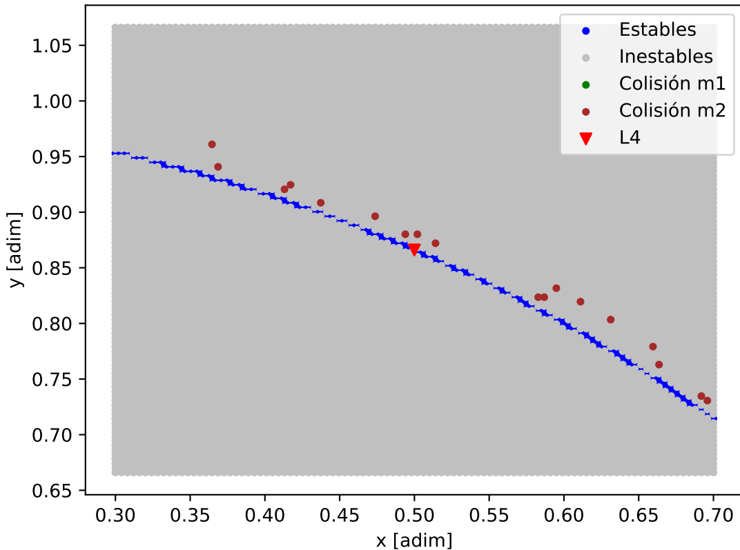
Mapa de estabilidad - K2-155
