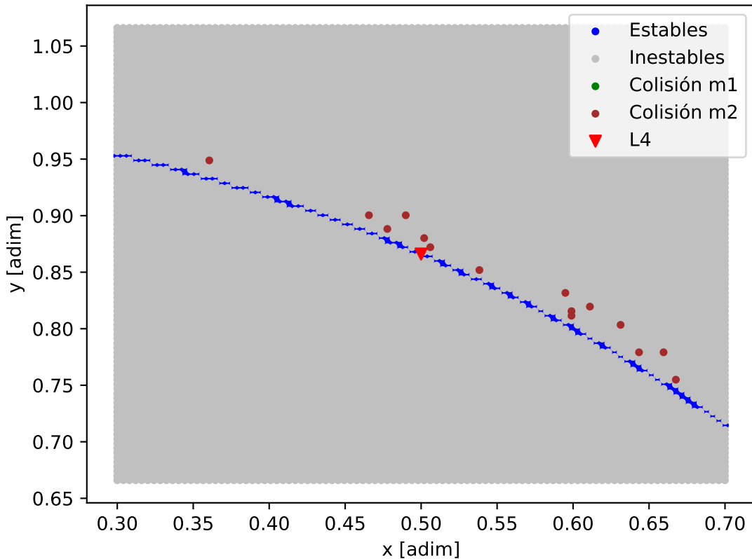
Mapa de estabilidad - K2-5
