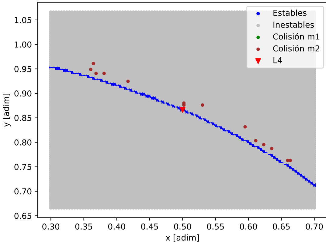
Mapa de estabilidad - K2-8
