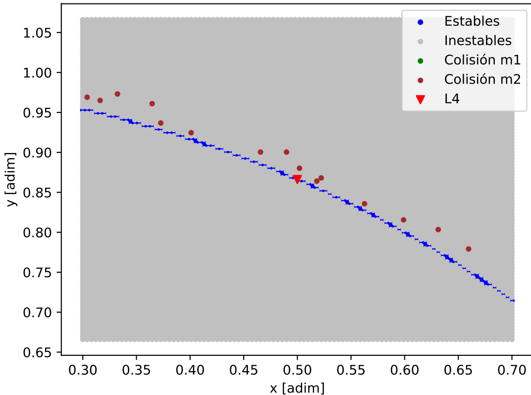
Mapa de estabilidad - Kepler-80
