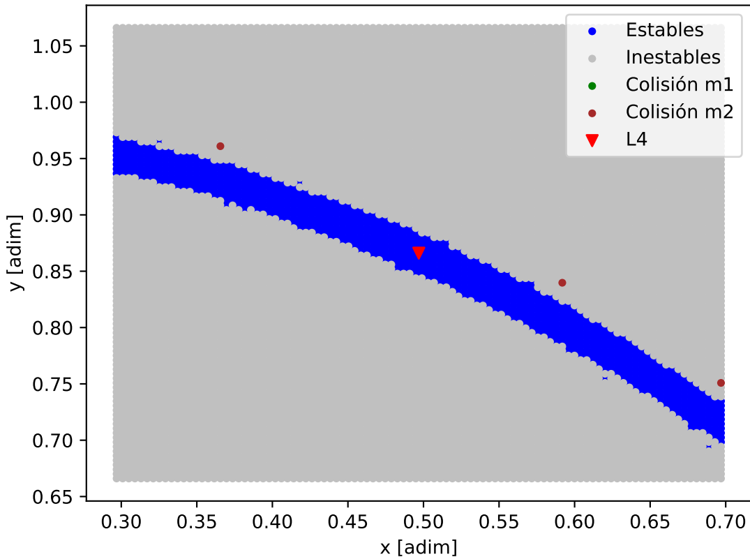
Mapa de estabilidad - PDS_70
