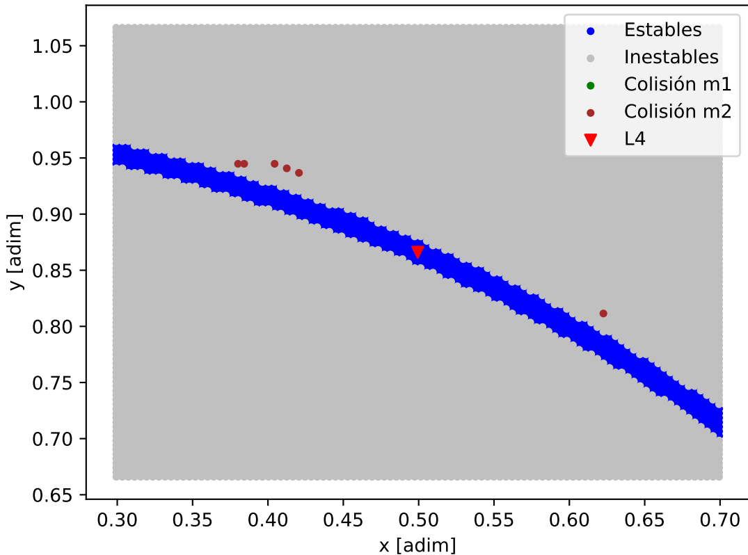
Mapa de estabilidad - HD_13908
