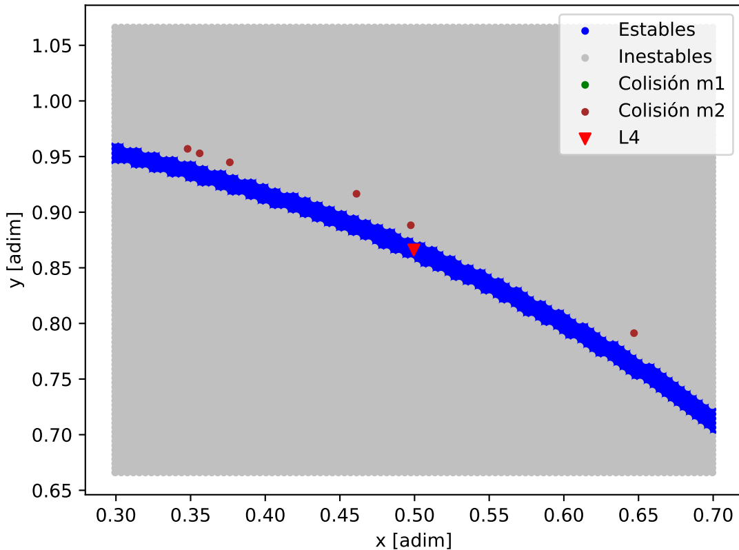
Mapa de estabilidad - TOI-1670
