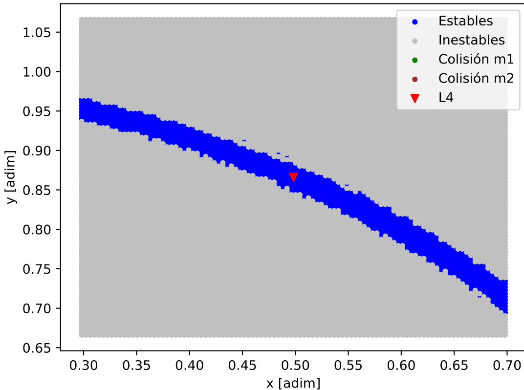
Mapa de estabilidad - TOI-4562
