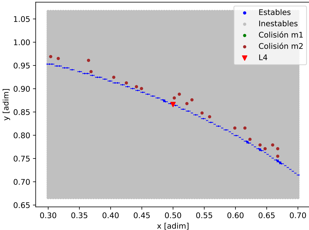
Mapa de estabilidad - TOI-1238
