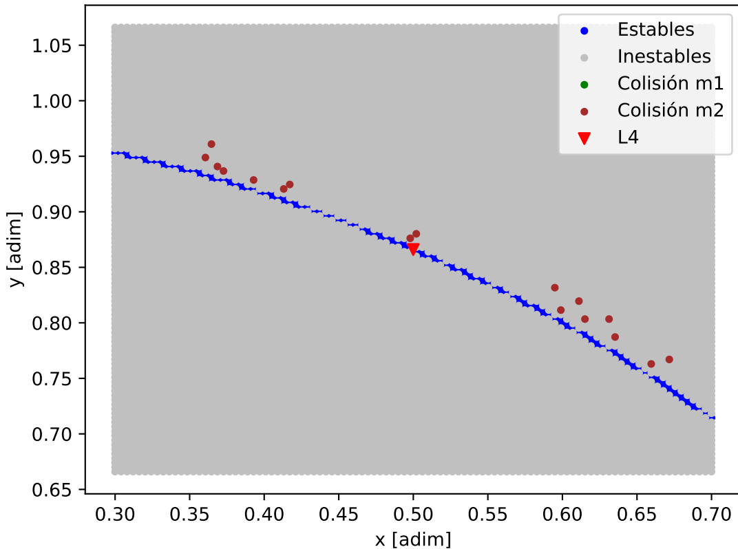
Mapa de estabilidad - TOI-2134
