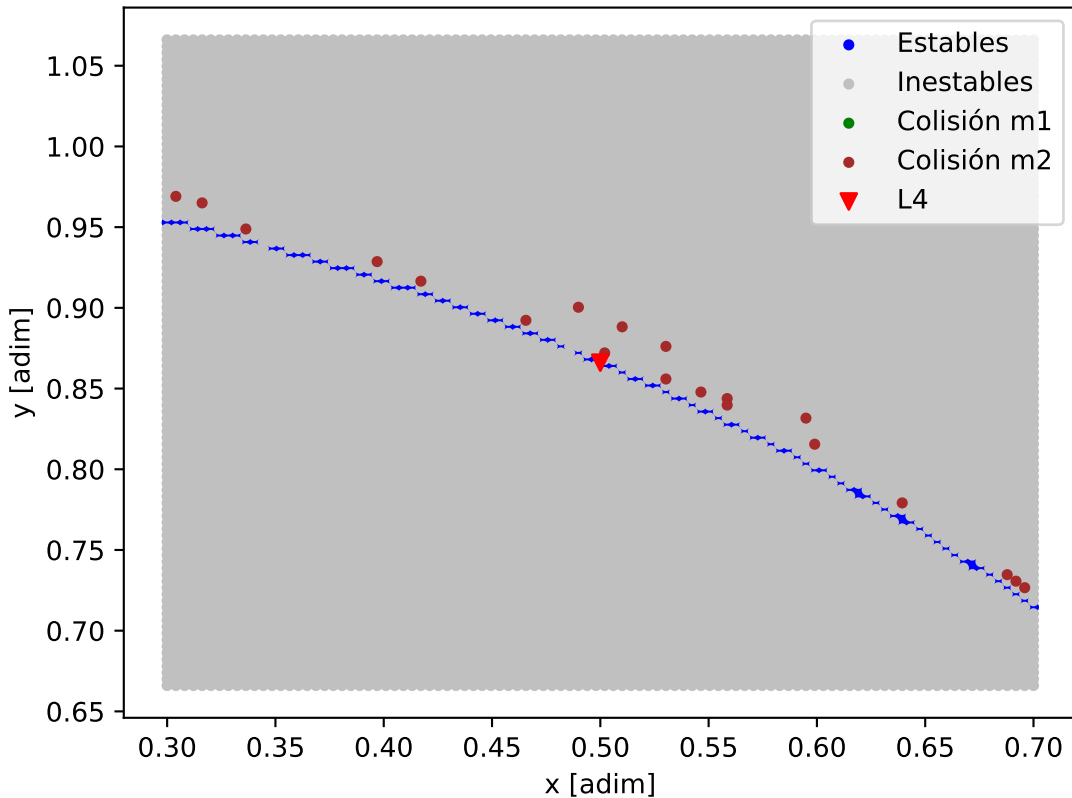
Mapa de estabilidad - TOI-286
