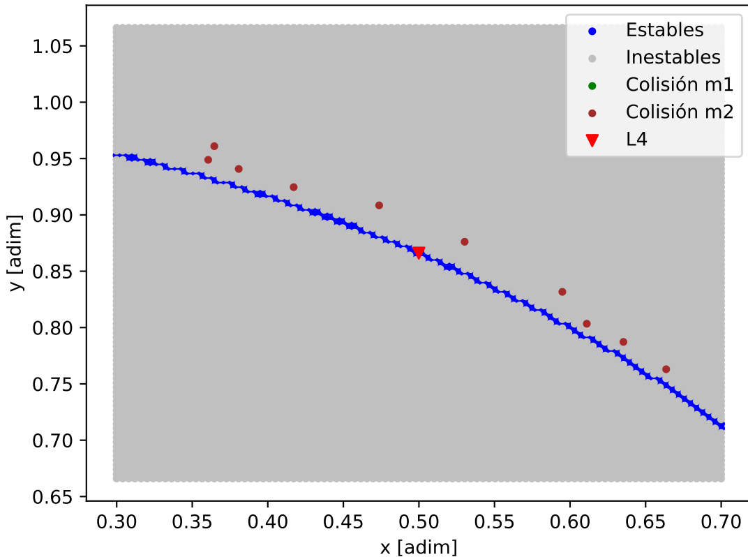
Mapa de estabilidad - TOI-4311
