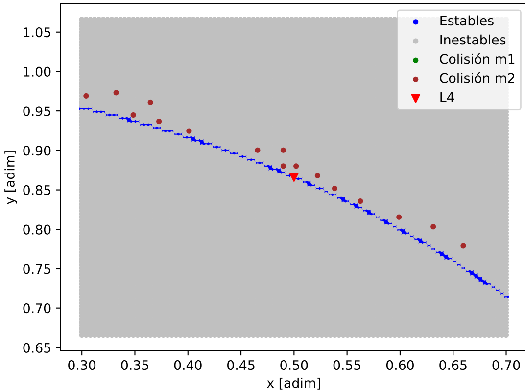
Mapa de estabilidad - TOI-4504
