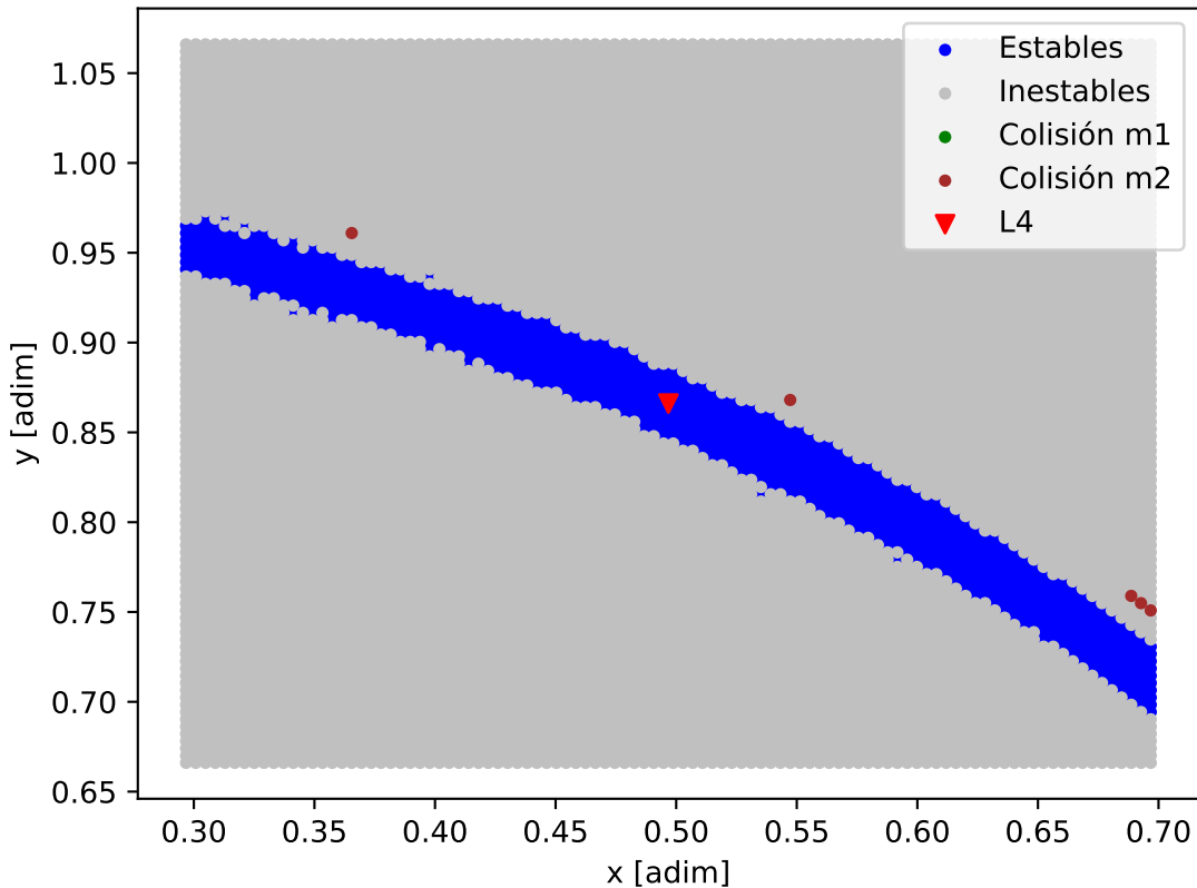
Mapa de estabilidad - TOI-4600
