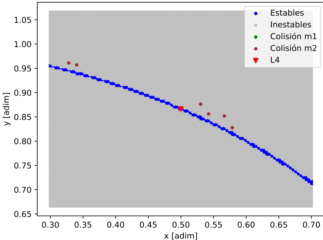
Mapa de estabilidad - TOI-880
