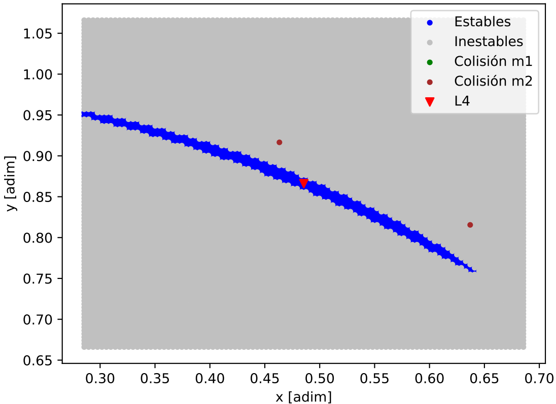
Mapa de estabilidad - TOI-969
