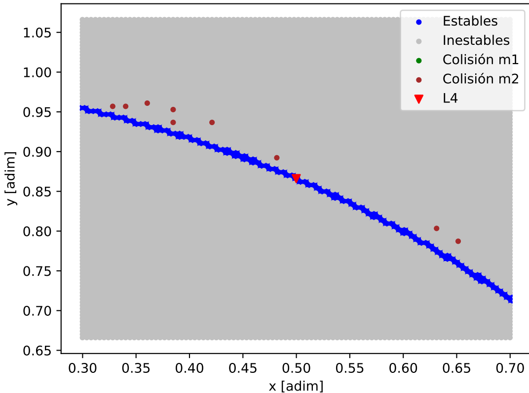
Mapa de estabilidad - WASP-107
