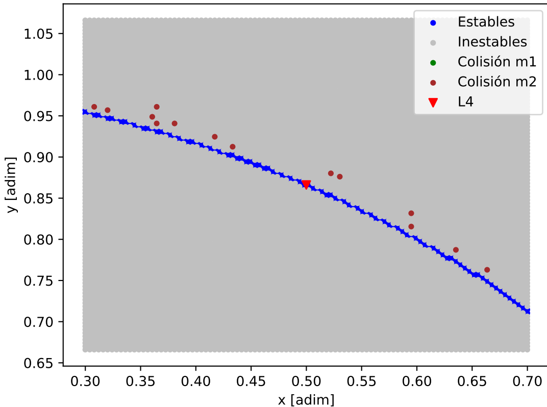
Mapa de estabilidad - WASP-84
