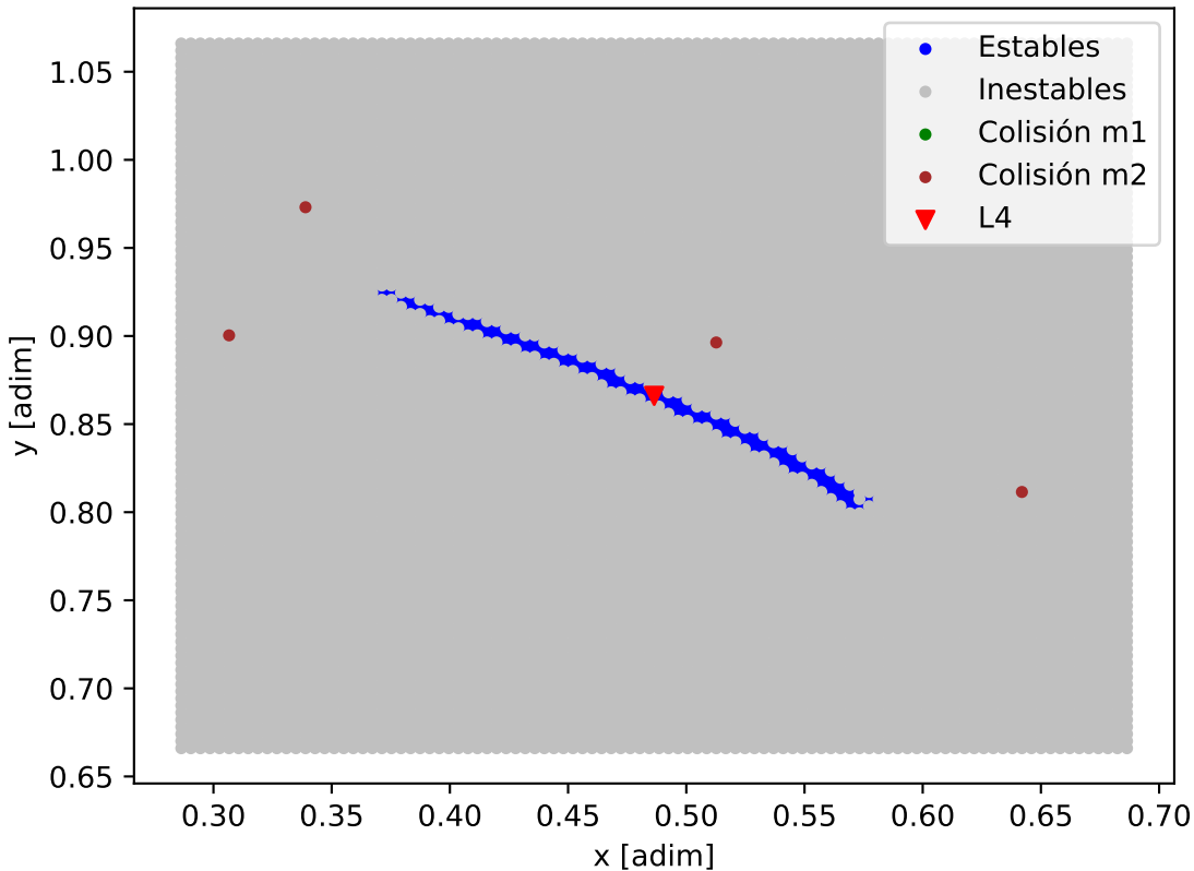
Mapa de estabilidad - WISPIT_1
