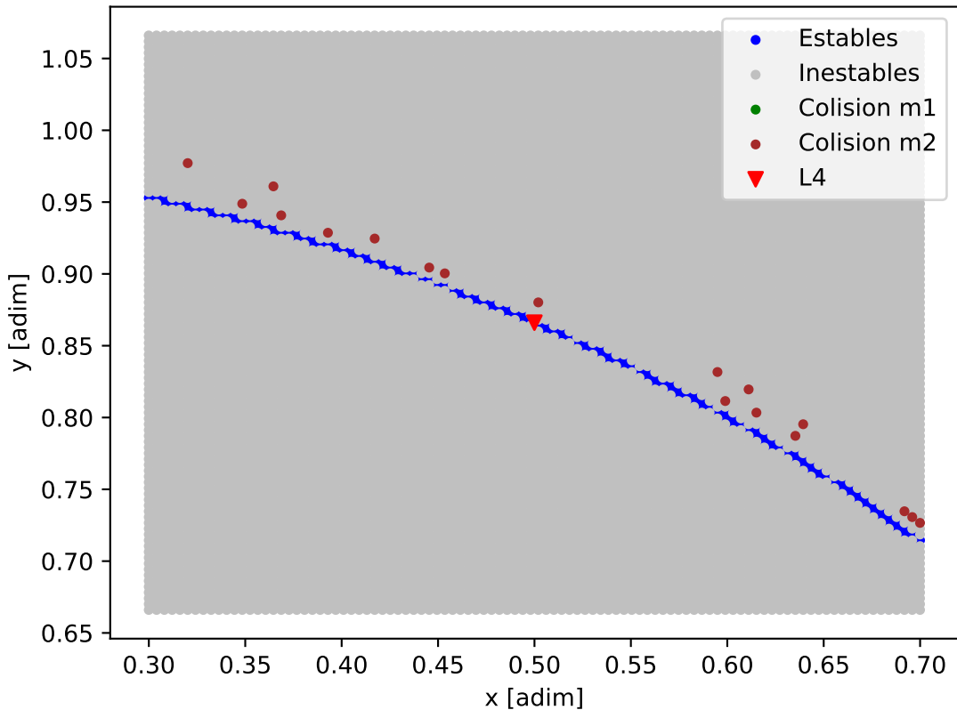
Mapa de estabilidad - 55_Cnc_B
