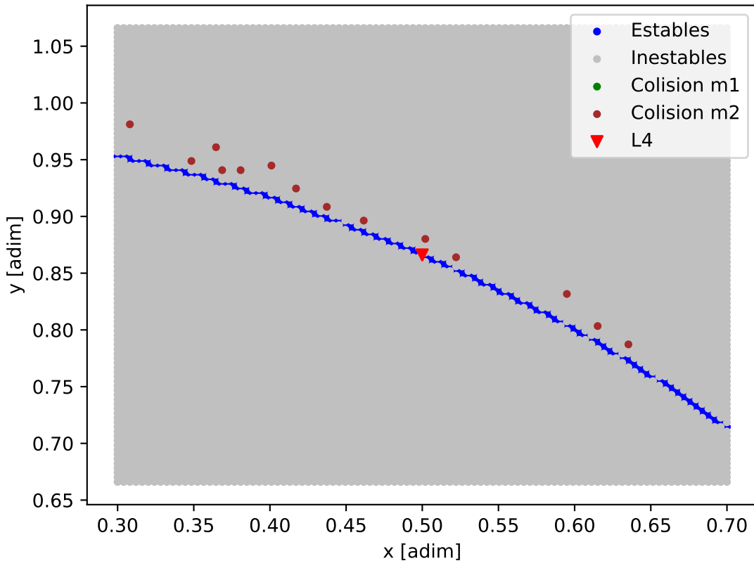
Mapa de estabilidad - AU_Mic
