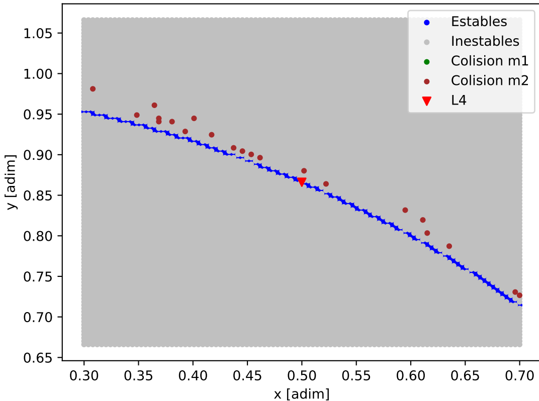
Mapa de estabilidad - GJ_1061
