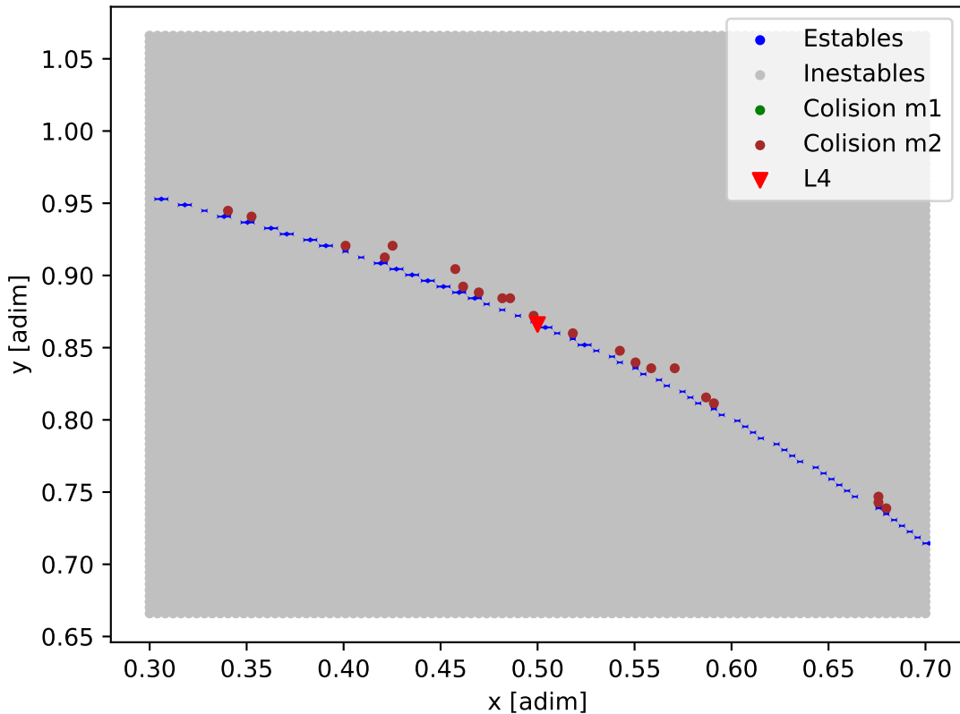
Mapa de estabilidad - GJ_367
