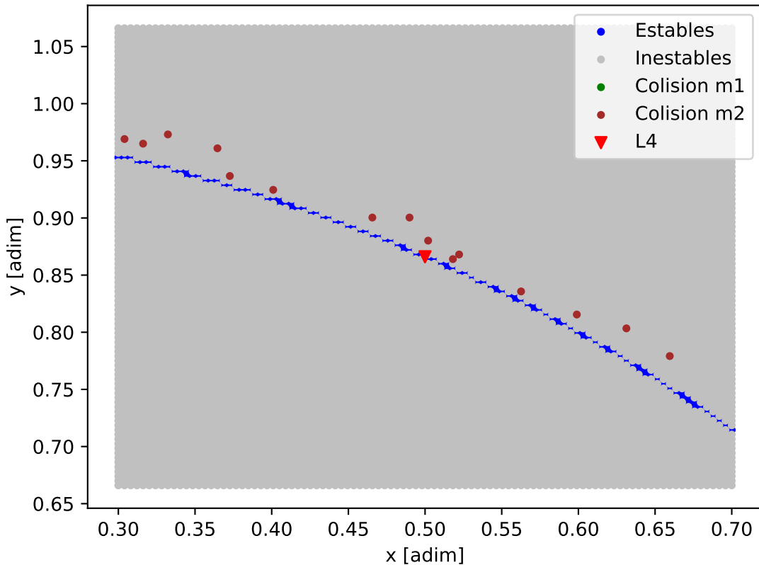
Mapa de estabilidad - GJ_581
