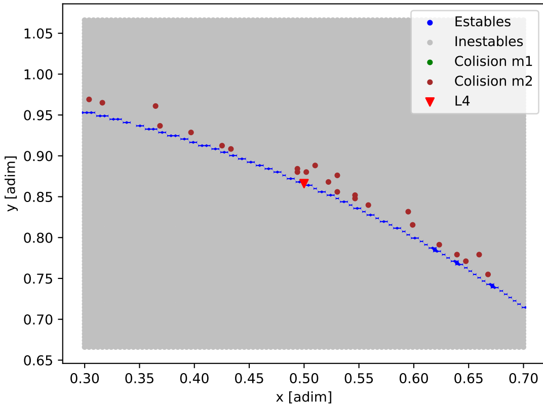
Mapa de estabilidad - GJ_676_A
