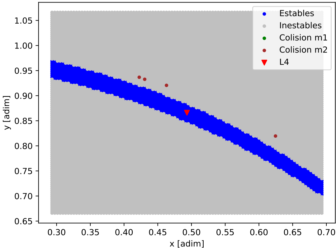
Mapa de estabilidad - GJ_876
