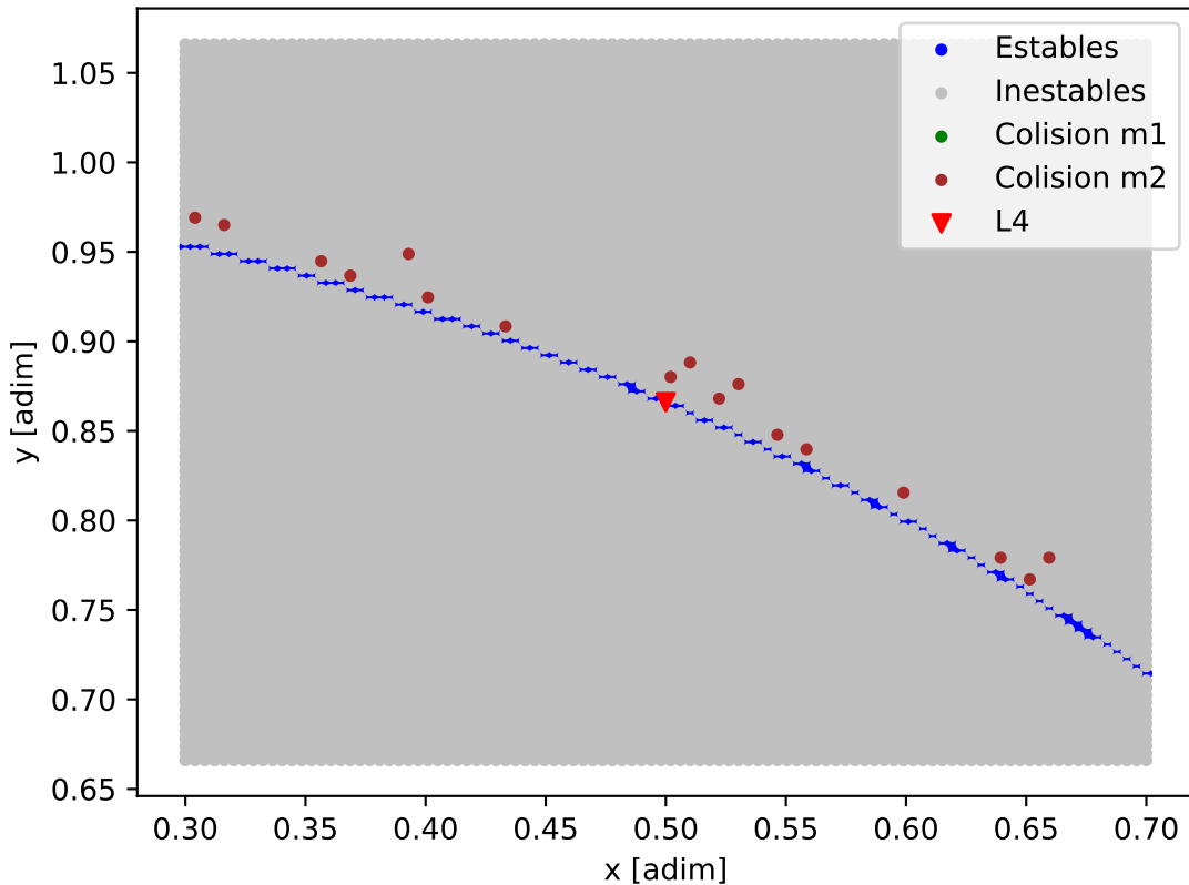
Mapa de estabilidad - K2-133
