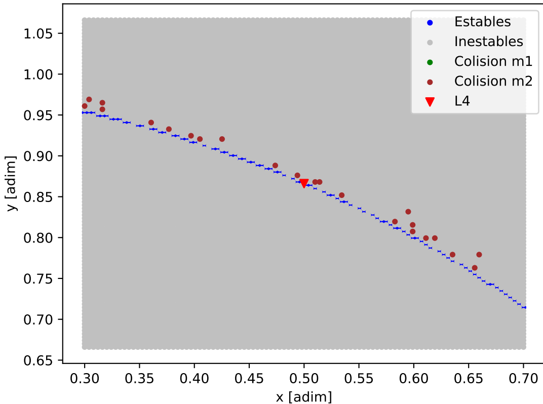
Mapa de estabilidad - K2-239
