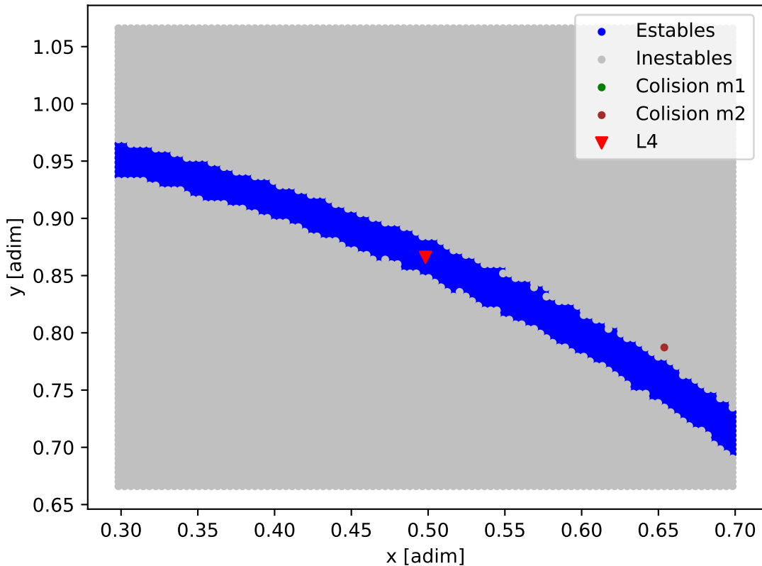
Mapa de estabilidad - KMT-2021-BLG-1077L
