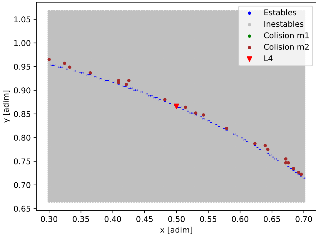
Mapa de estabilidad - Kepler-138
