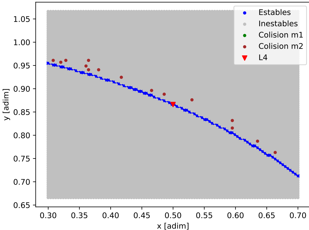
Mapa de estabilidad - Kepler-159
