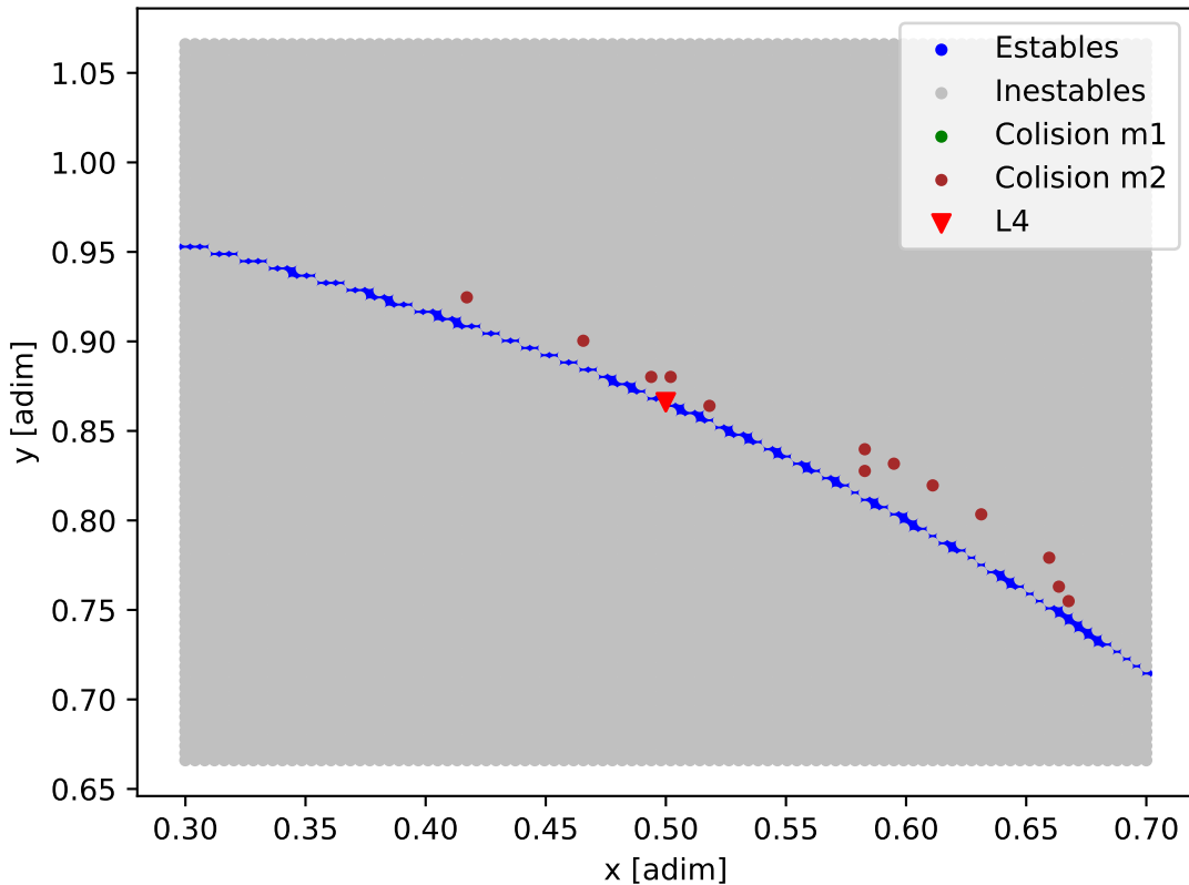
Mapa de estabilidad - Kepler-296
