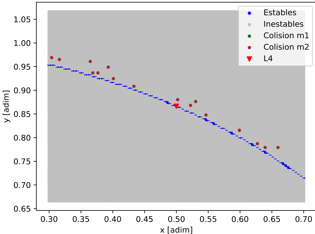
Mapa de estabilidad - Kepler-32
