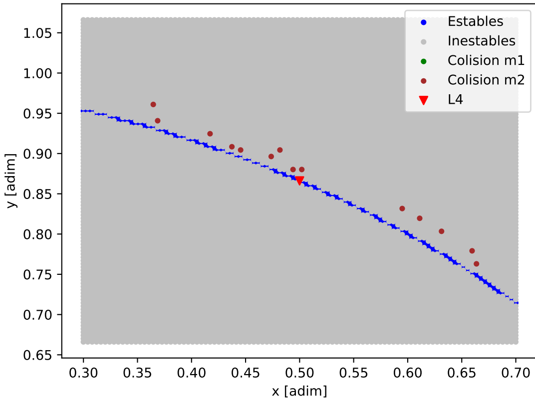
Mapa de estabilidad - Kepler-446
