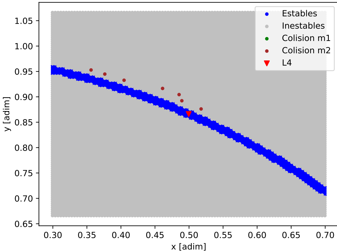
Mapa de estabilidad - Kepler-52
