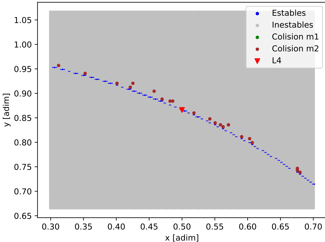
Mapa de estabilidad - Kepler-54
