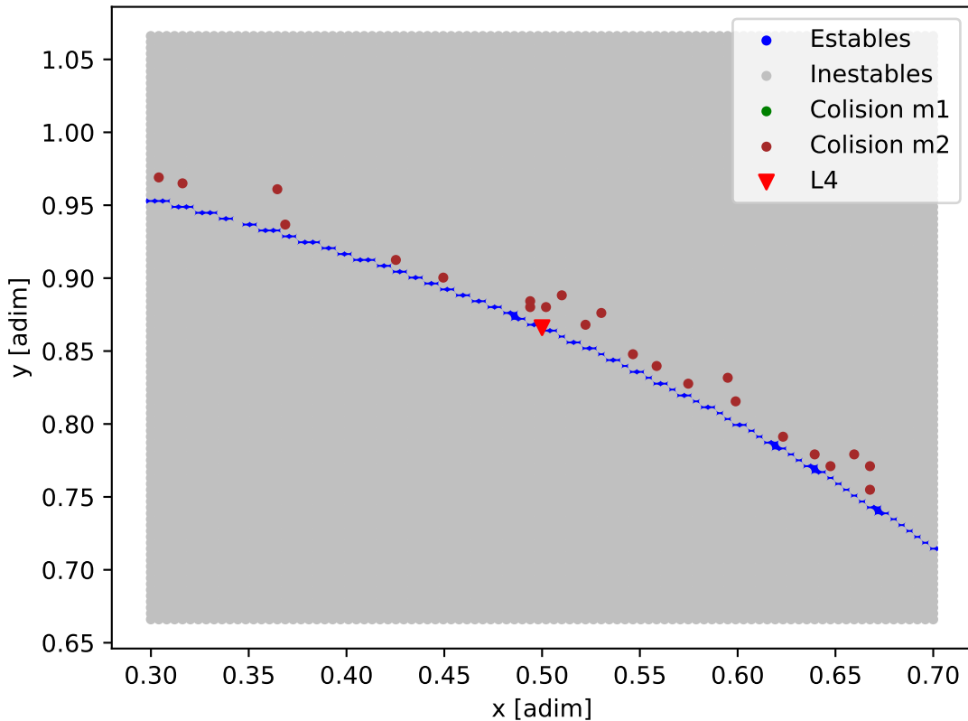
Mapa de estabilidad - Kepler-83
