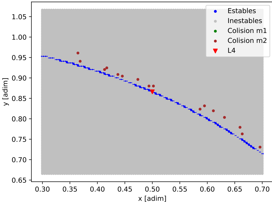
Mapa de estabilidad - LHS_1903
