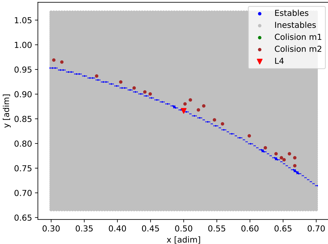
Mapa de estabilidad - LTT_3780
