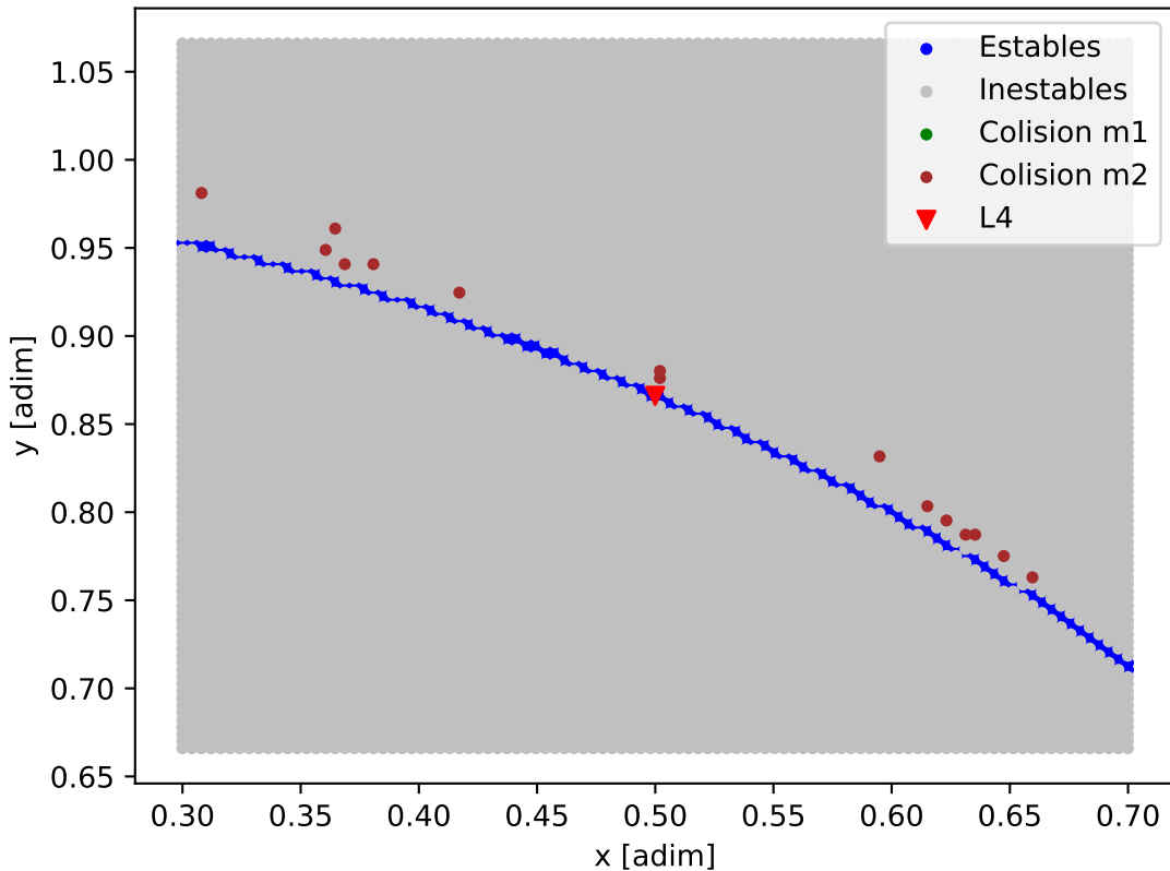
Mapa de estabilidad - TOI-1470
