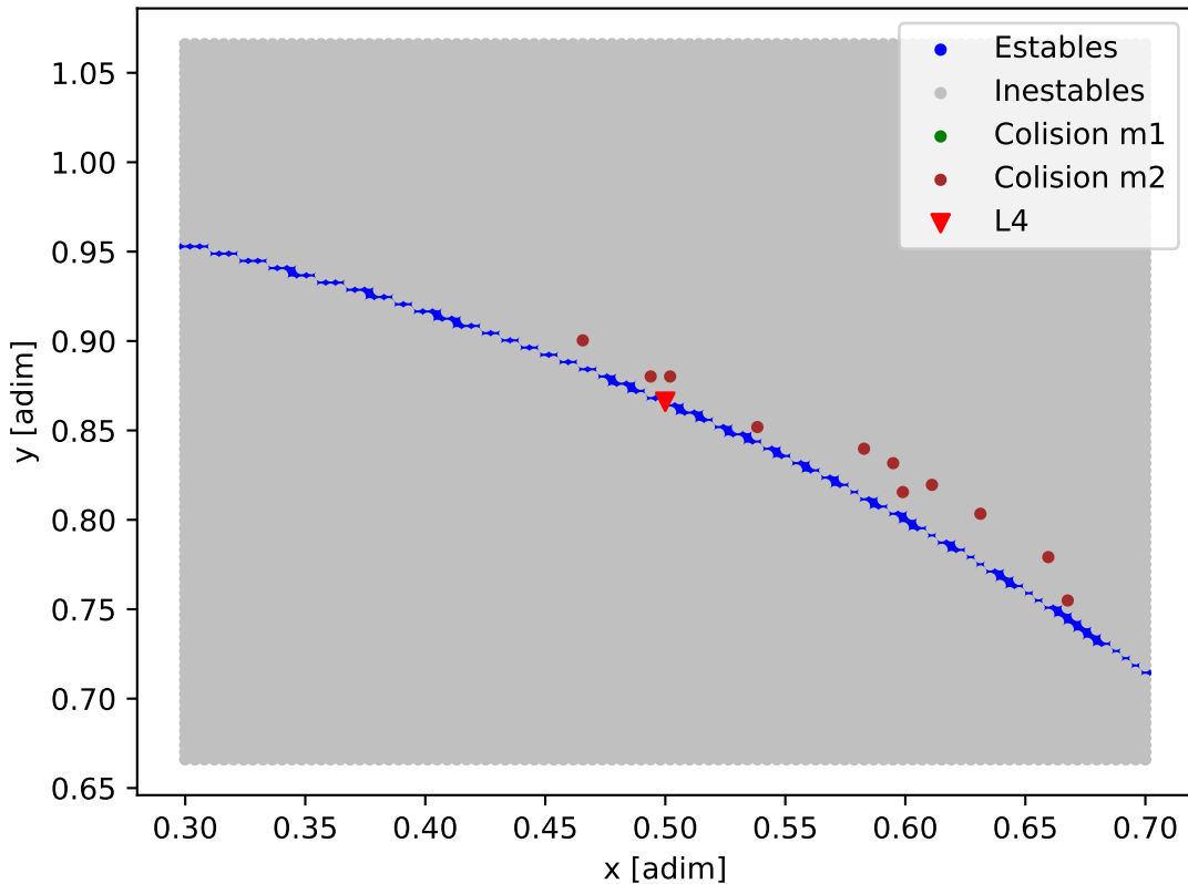
Mapa de estabilidad - TOI-1634
