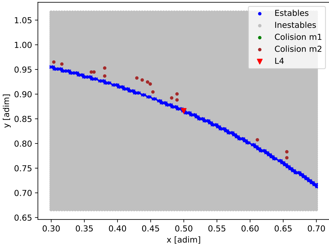
Mapa de estabilidad - TOI-2267_B
