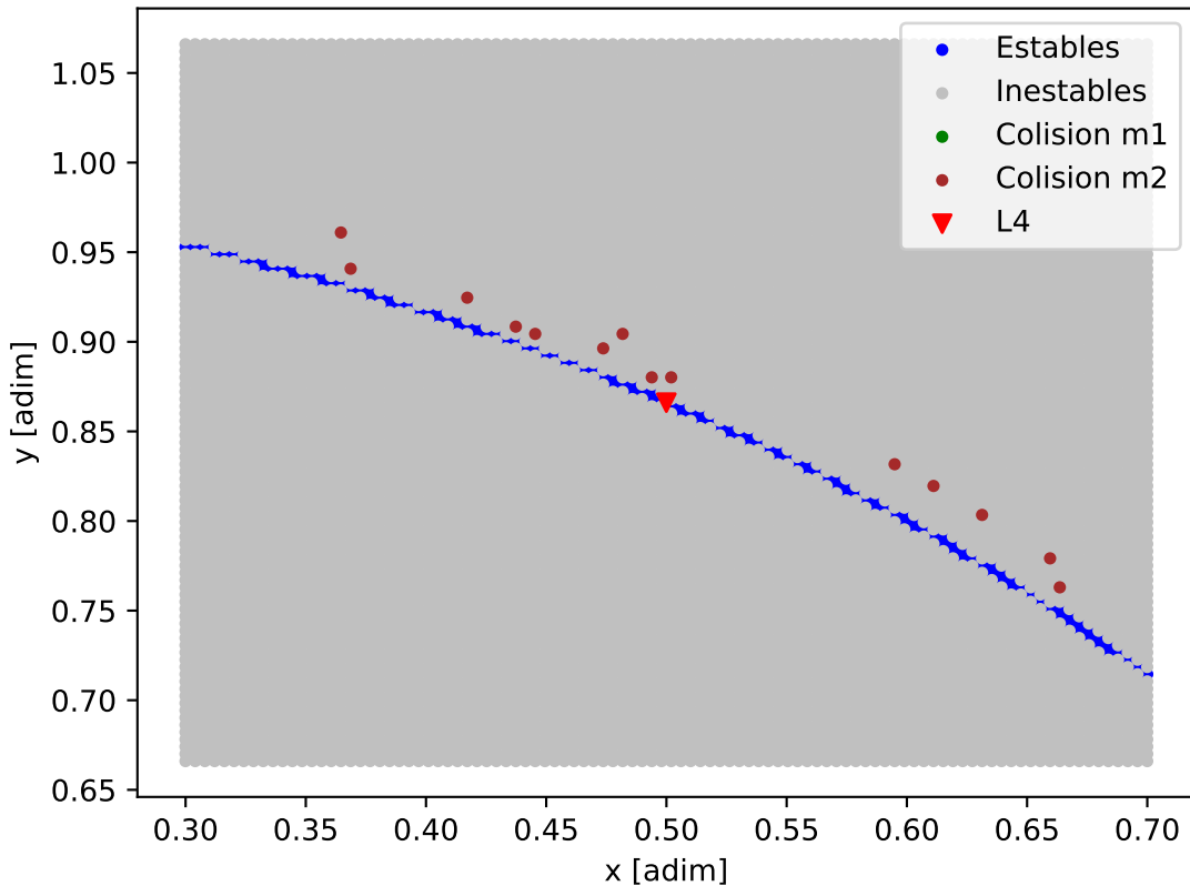
Mapa de estabilidad - TOI-270
